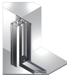
C: Montage hinter der Mauerlaibung mit schmalen Montageprofil
