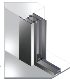
E: Montage innerhalb der Mauerlaibung mit innerer Abdeckleiste
