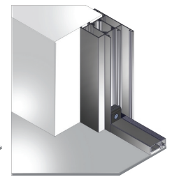
F: Montage innerhalb der Mauerlaibung mit äußerer Abdeckleiste
