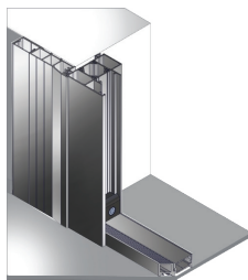
B: Montage innerhalb der Mauerlaibung mit breitem Montageprofil
